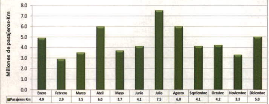
Pasajeros-Km Mensuales 2011
