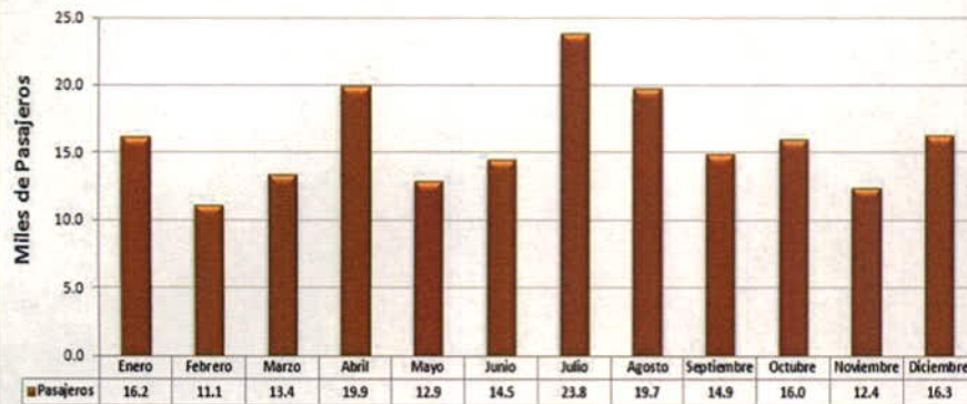
Pasajeros Mensuales 2011
